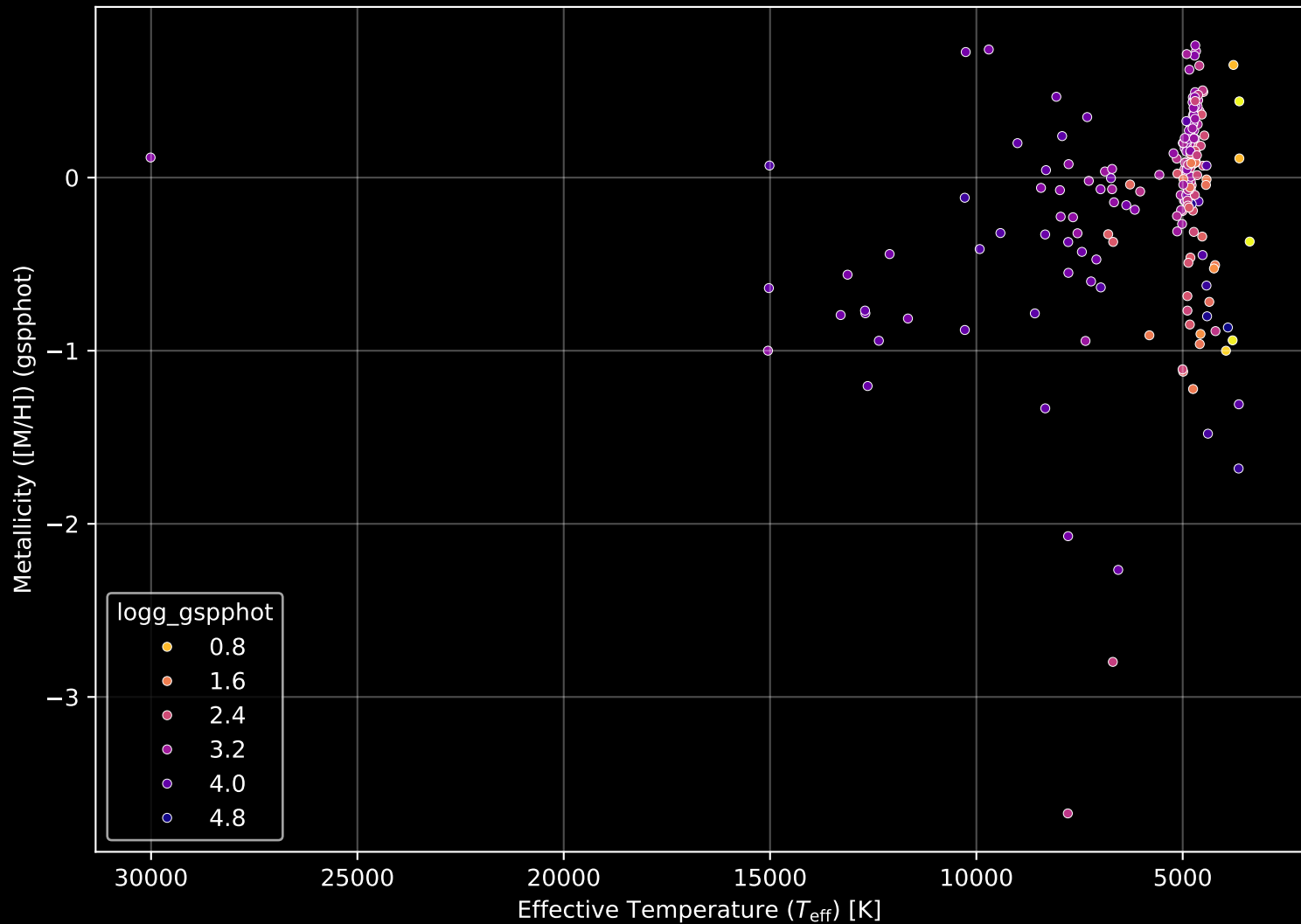
APOGEE DR17 Field: [049+00] Stellar Population Parameters (n= 209)
